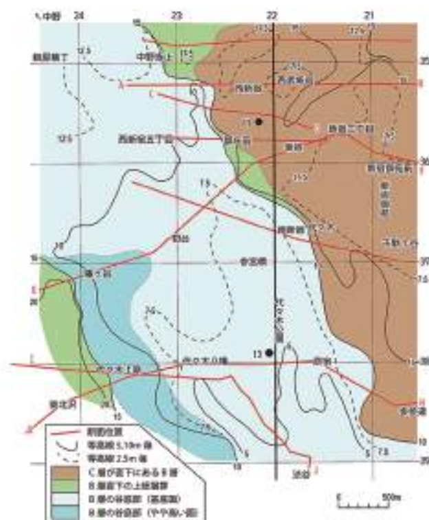
図7 代々木-高輪埋没谷の基底地形とC層の分布
