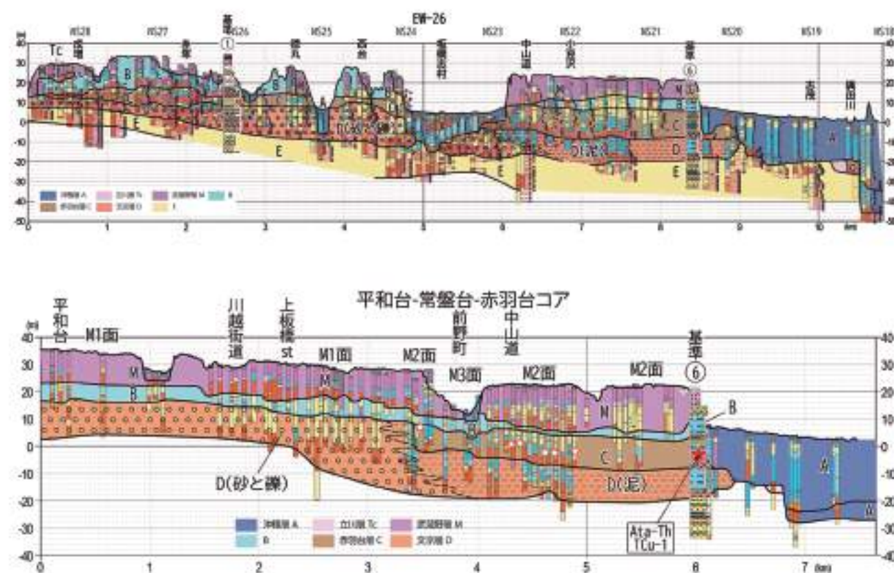
図19 D層に着目した武蔵野台地最北部の断面図 EW-26断面、平和台-常盤台-赤羽台断面図
