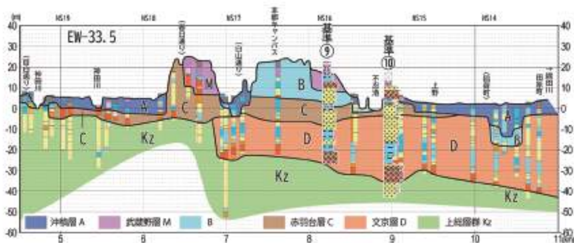
図13 小石川-本郷-上野地区の断面 (EW-33.5断面図)
