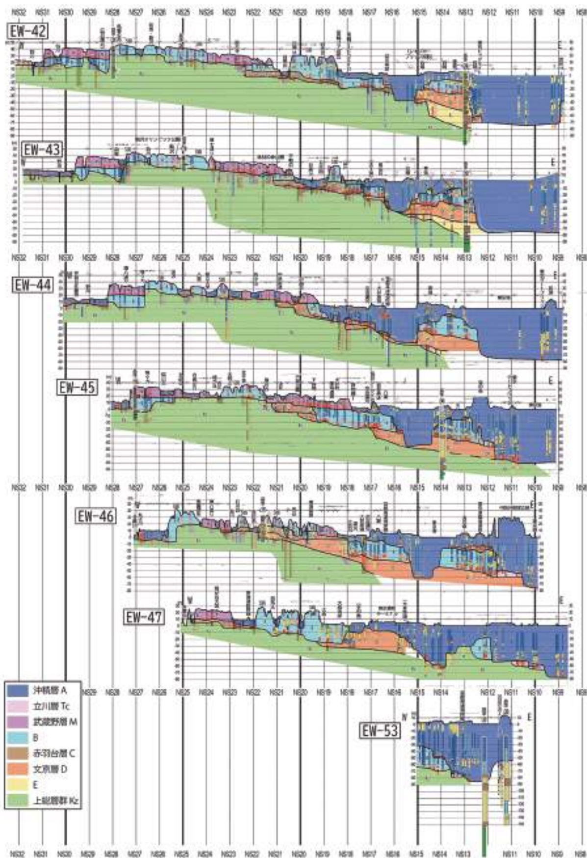
図5-1-3 EW断面図
