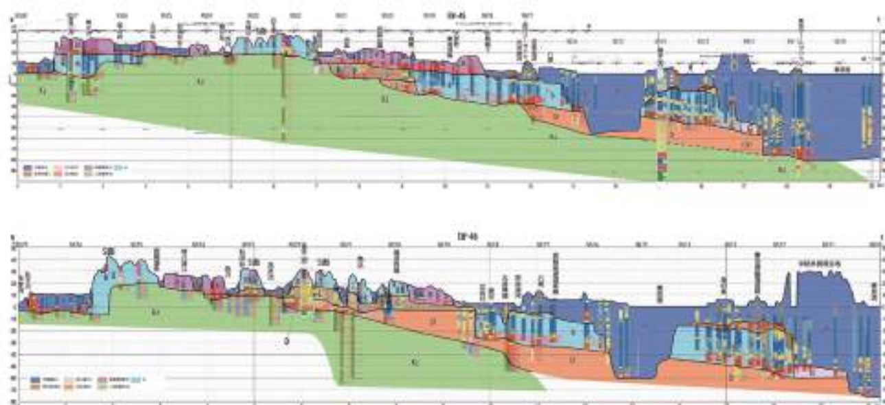
図22 臨海部を代表する断面図 (EW-45,EW-46)
