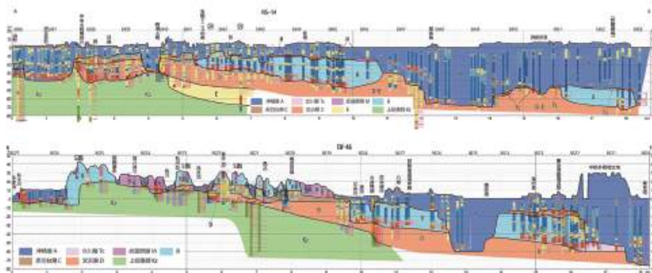
図15 NS-14断面図とEW-46断面図
