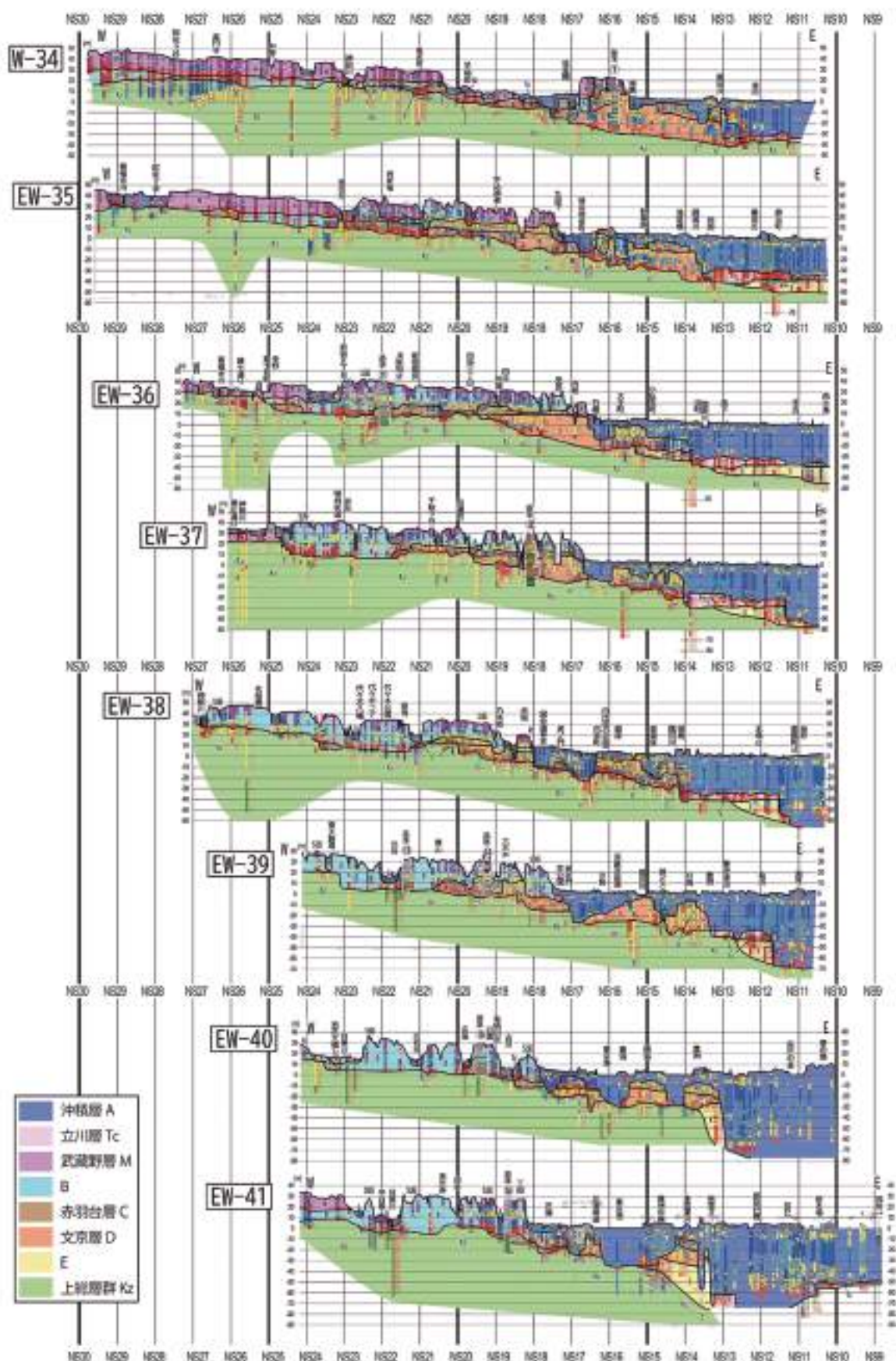
図5-1-2 EW断面図
