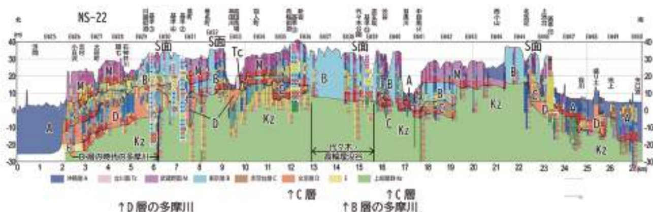
図9 南北断面におけるB層、C層の埋層 (NS-22断面、縦軸3倍強調)
