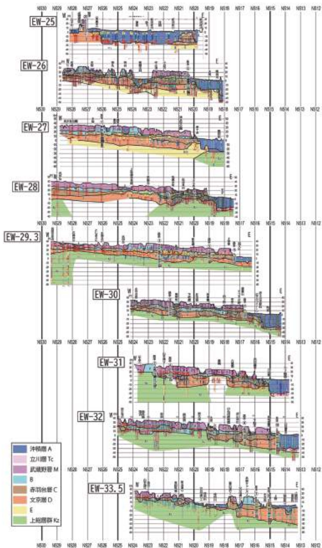
図5-1-1 EW断面図
