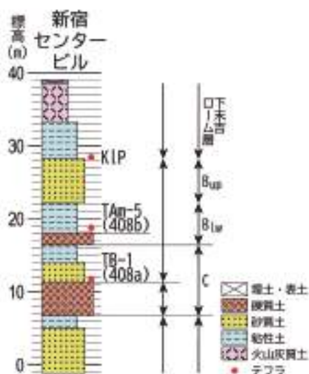
図4 新宿センタービル柱状図 [No.11, 図2] (杉原, 1979に基づく)
