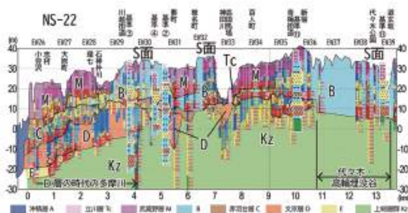
図18 上総層群の高まりとD層のV字谷(NS-22断面図、縦軸3倍強調)
