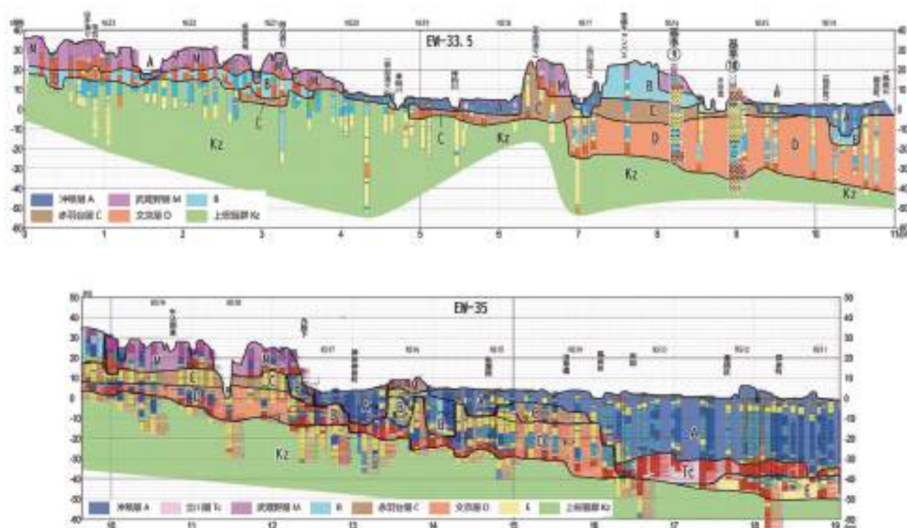
図21 D層に着目した武蔵野台地中北部の断面図：EW-33.5とEW-35断面アップ
