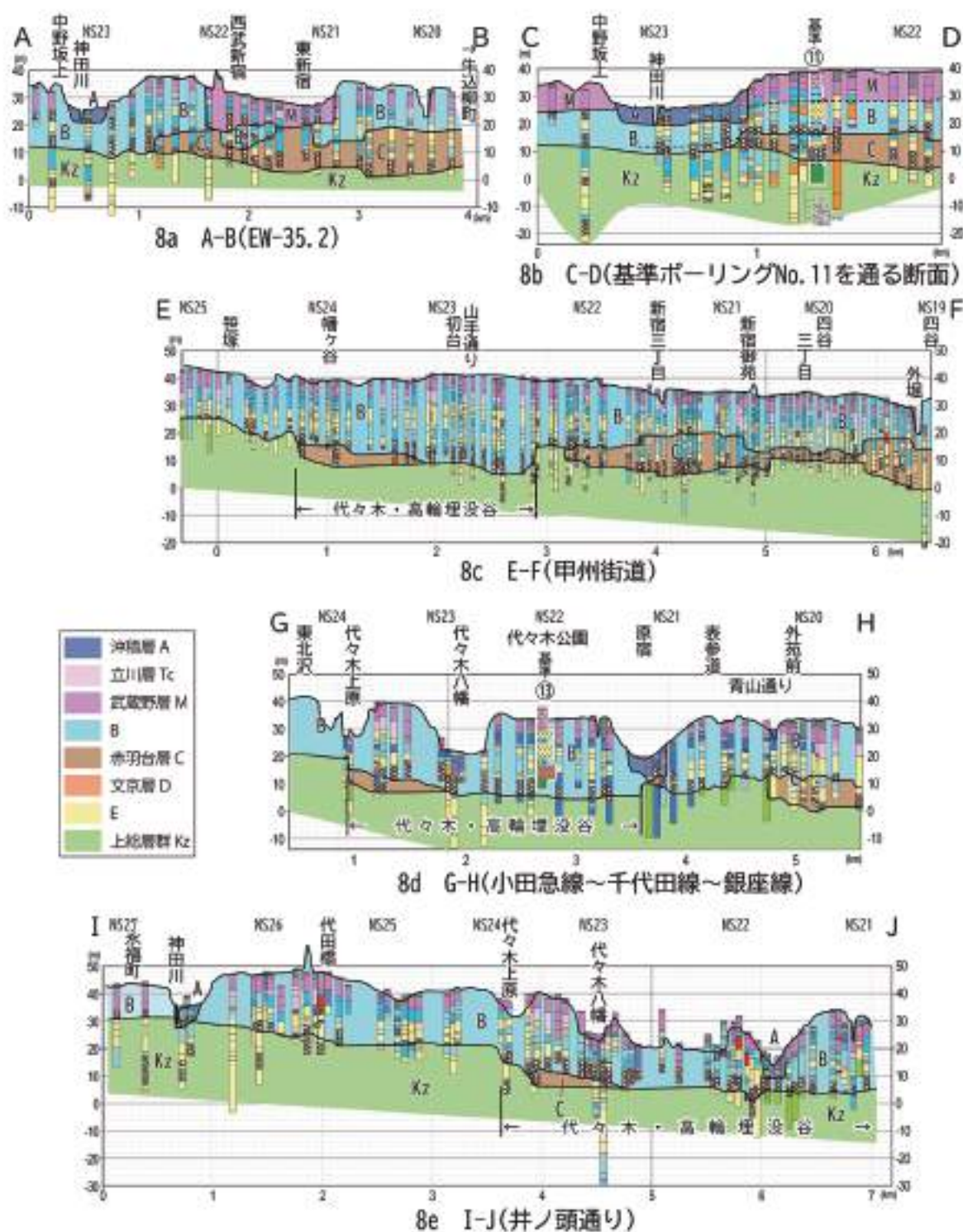
図8 代々木-高輪埋没谷の地質断面図 柱状図の右側のバーはN値を示す
