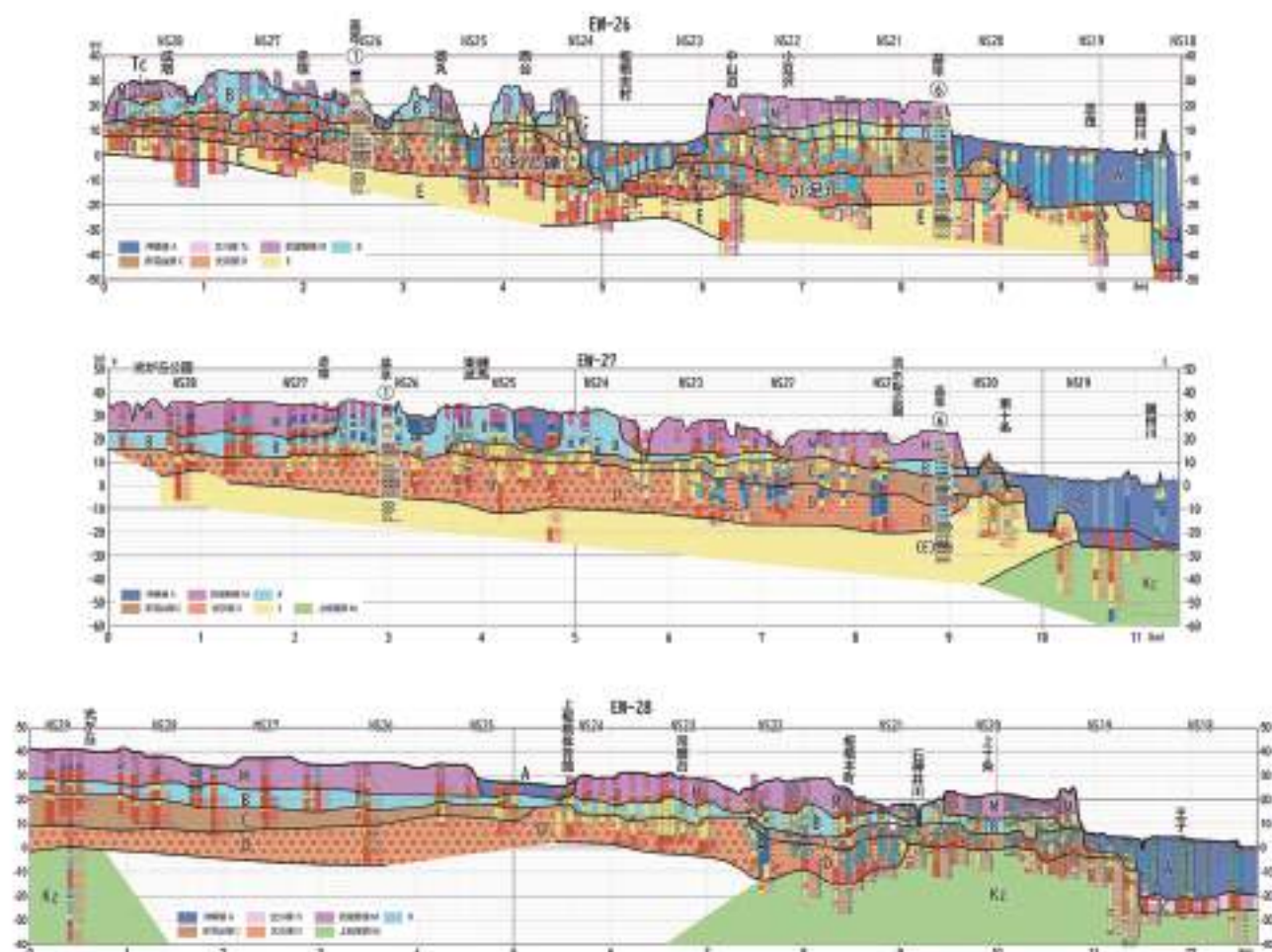
図20 D層の現状地とつながる部分 (D1-F) の断面図 (EW-26, EW-27, EW-28)
