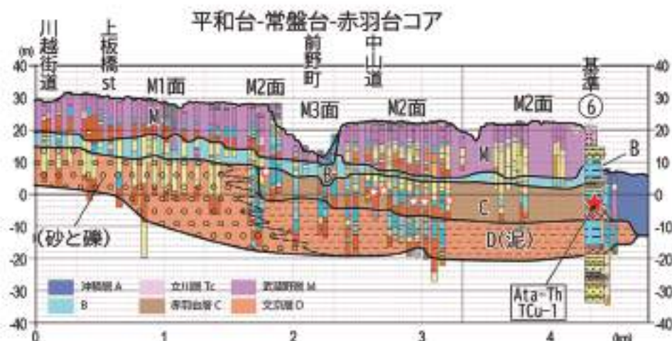
図12 平和台-常盤台-赤羽台断面図
